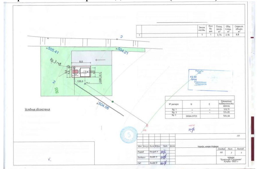
Чертёж генеральный план (ГП)
