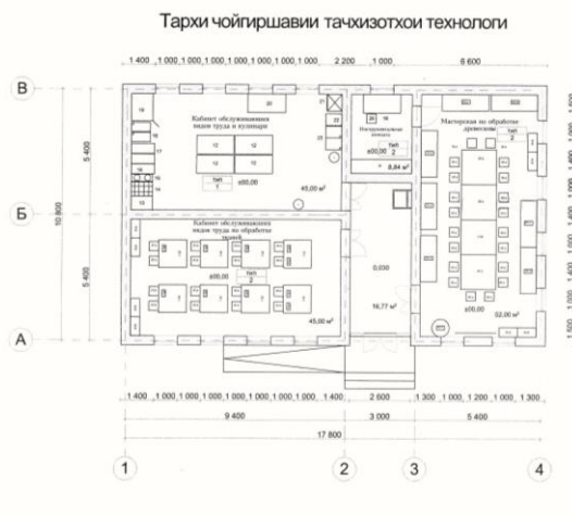
План расстановки технологического оборудования
