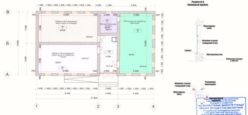
Фото: План технологических классов
