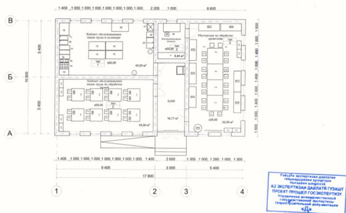
Фото: План расстановки оборудования в технологических классах
