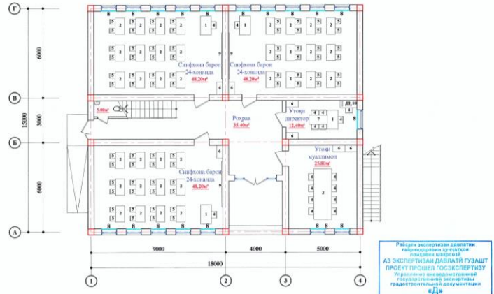
План технологического оборудования второго этажа
