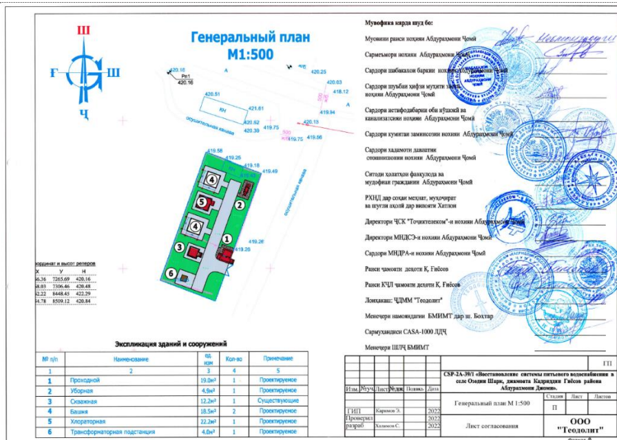
Чертёж: Генеральный план (ГП для села Озодии шарк).
