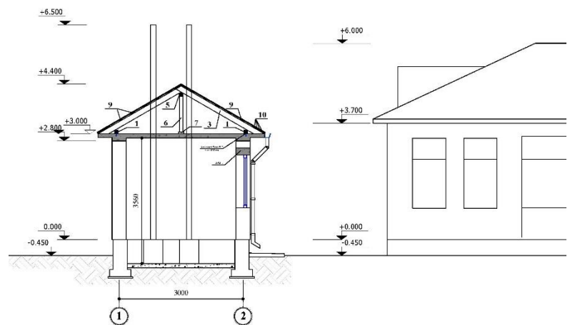
Эскиз основного здания и котельная
