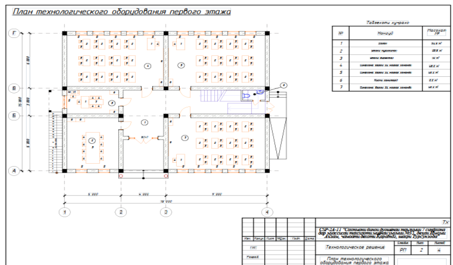
План 1-го этажа учебного корпуса в селе Халкаруд
