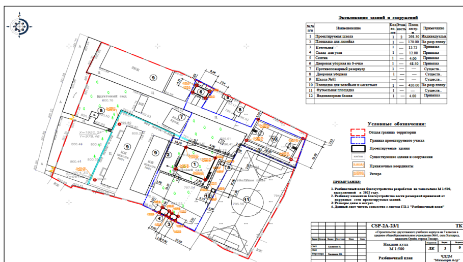
Чертёж: Генеральный план (ГП).
