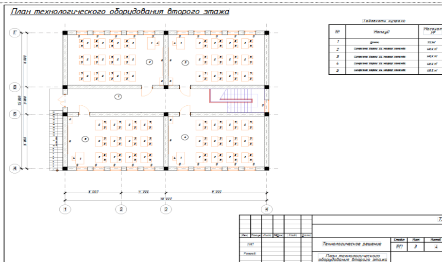
План 2-го этажа учебного корпуса в селе Халкаруд
