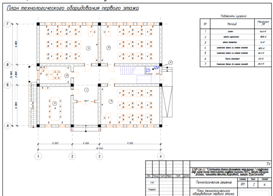
План 1-го этажа учебного корпуса в селе Чинор
