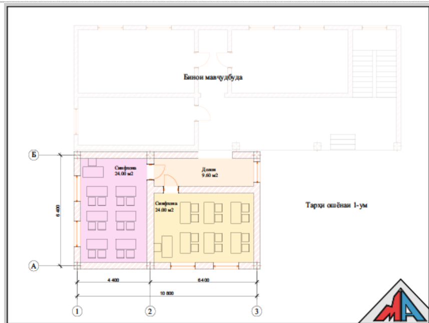
План 1-го этажа учебного корпуса в селе Вахдат
