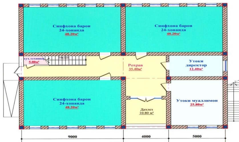
План 1-го этажа учебного корпуса в махалле Какир
