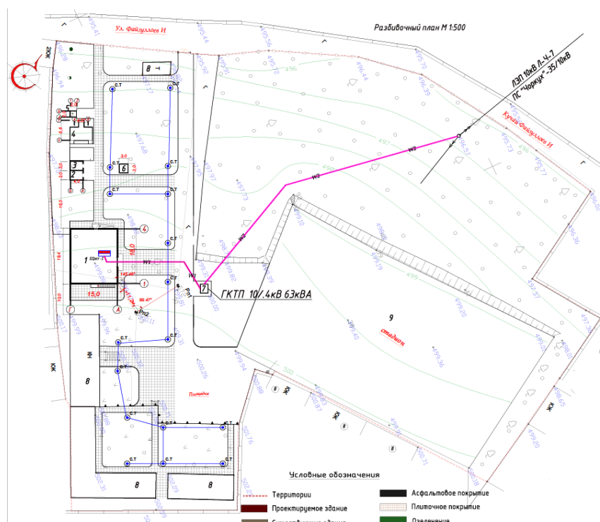
Чертёж: Генеральный план (ГП).
